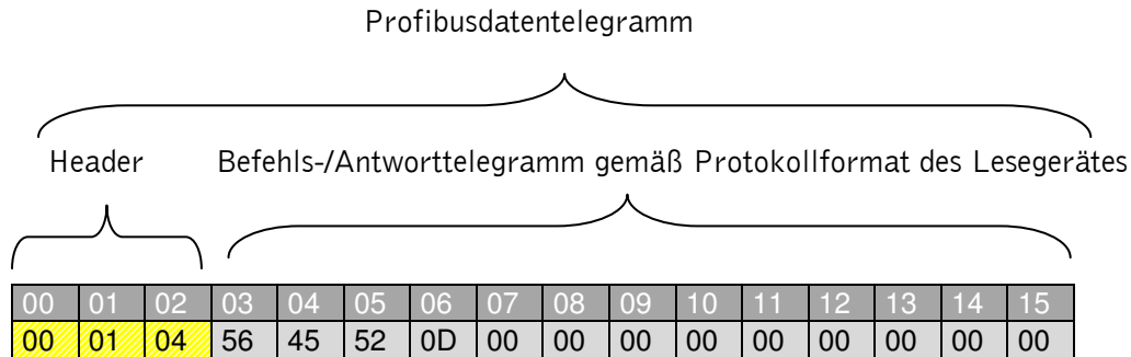
Abbildung 0-1 Datenbereich des Profibusdatentelegramms
